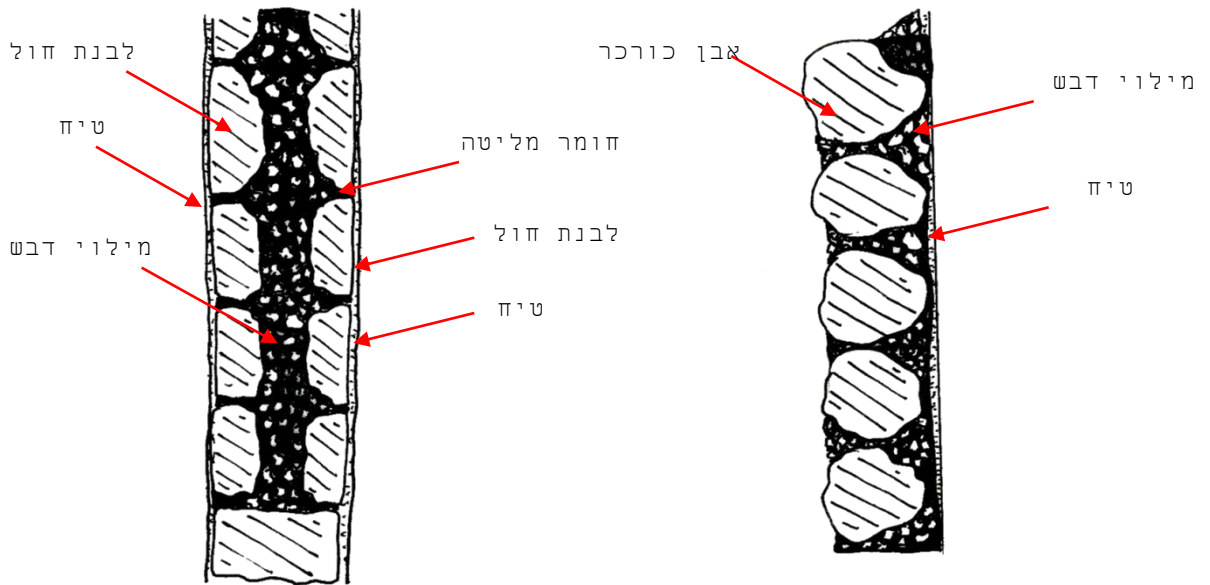
חתך עקרוני של קירות מבנה הח'אן ובית הבאר משנת 1928
