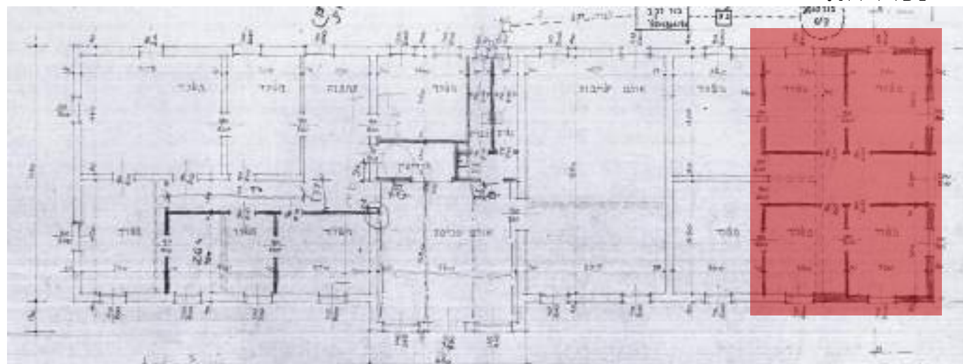
מבנה הח'אן 1957, הוספת אגף וסגירת 4 דלתות בחזית המבנה
