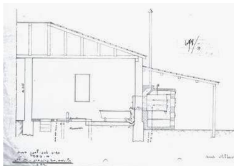
1929- חתך ה-ו חתך באזור התנוור החיצוני, האמבטיות והמקווה
