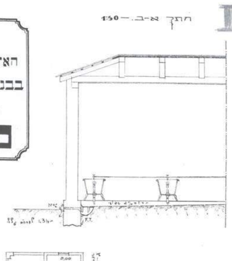
1929- חתך א-ב, חתך באזור חדרי אמבטיות
