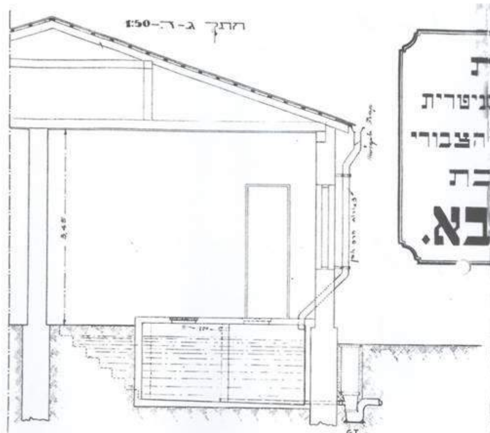
1929- חתך ג-ד חתך באזור התנוור המקווה
