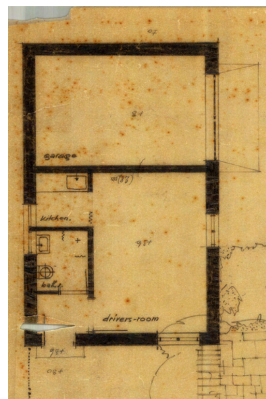
קטע מתוכנית רכטר לוילה המראה את בית הנהג (מקור: ארכיון רכטר, באדיבות אמנון רכטר)
