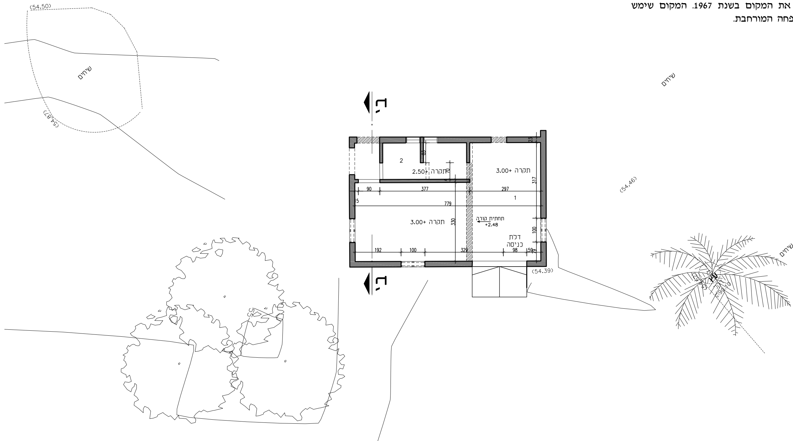
תוכנית קומת קרקע - מצב מקורי משוחזר - בית הנהג קנה מידה 1:100
